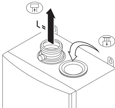
Afb.32 Open uitvoering
