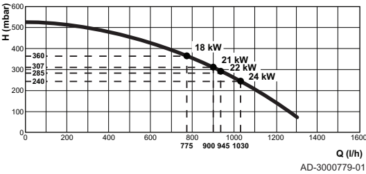
Afb.9 Restopvoerhoogte Avanta 28c
