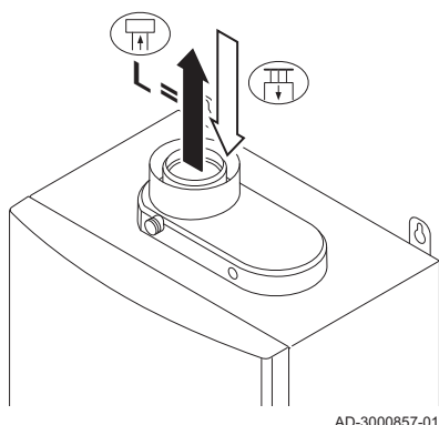
Afb.34 Gesloten uitvoering (concentrisch)
