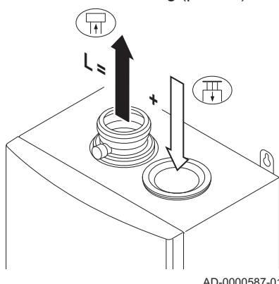
Afb.35 Gesloten uitvoering (parallel)
