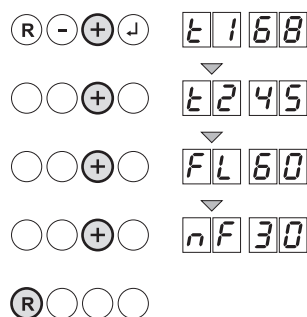
Afb.66 Uitlezen waarden
