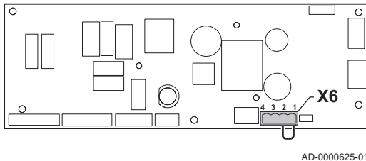
Afb.44 Blokkerende ingang
