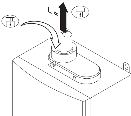
Afb.33 Open uitvoering
