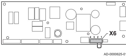
Afb.43 Aansluiten vorstthermostaat
