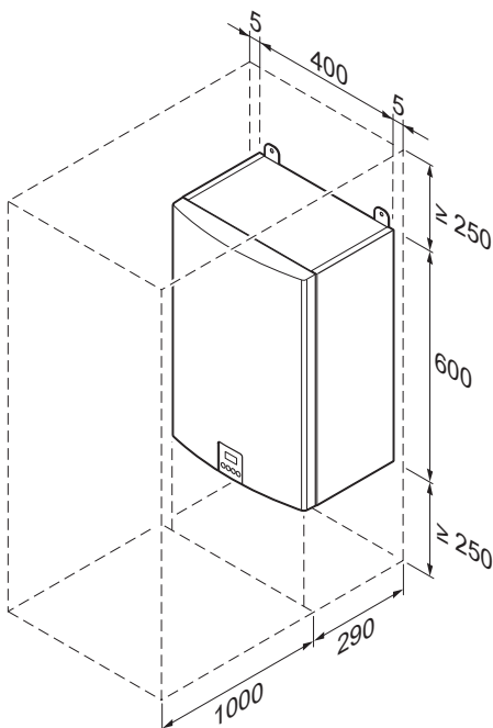
Afb.16 Montageruimte
