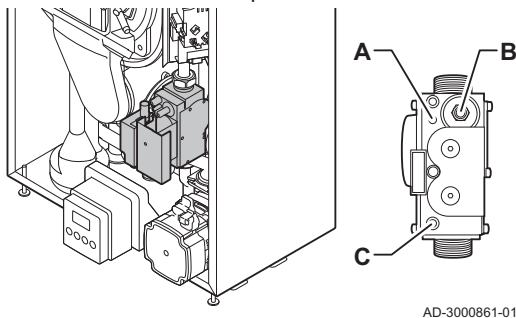
Afb.48 Gasblok meetpunt C
