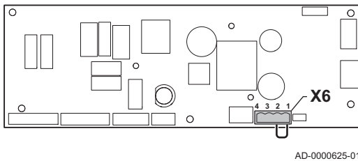
Afb.42 Aansluiten aan/uit thermostaat
