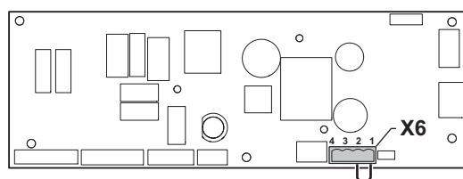
Afb.41 Aansluiten modulerende thermostaat
