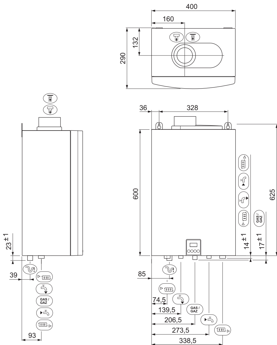
Afb.7 Afmetingen (concentrisch)
