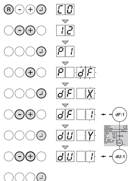
Afb.63 Fabrieksinstellingen terugzetten
