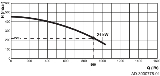
Afb.8 Restopvoerhoogte Avanta 24c
