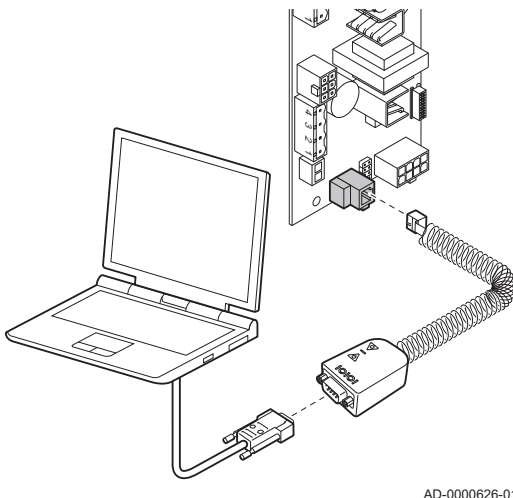
Afb.45 Aansluiten PC/laptop
