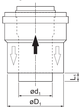
Afb.31 Afmetingen concentrische aansluiting
