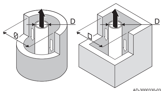
Afb.28 Minimale afmeting schacht of koker C 93
